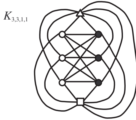
図 2.1: K_{3,3,1,1}
